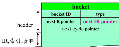
圖 4 封包的表頭
