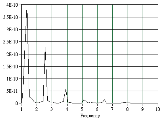
圖 4-2 頻譜圖
