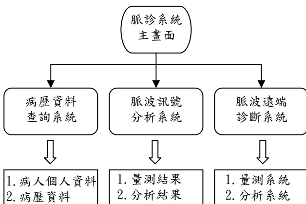
圖 3-1 軟體架構圖
