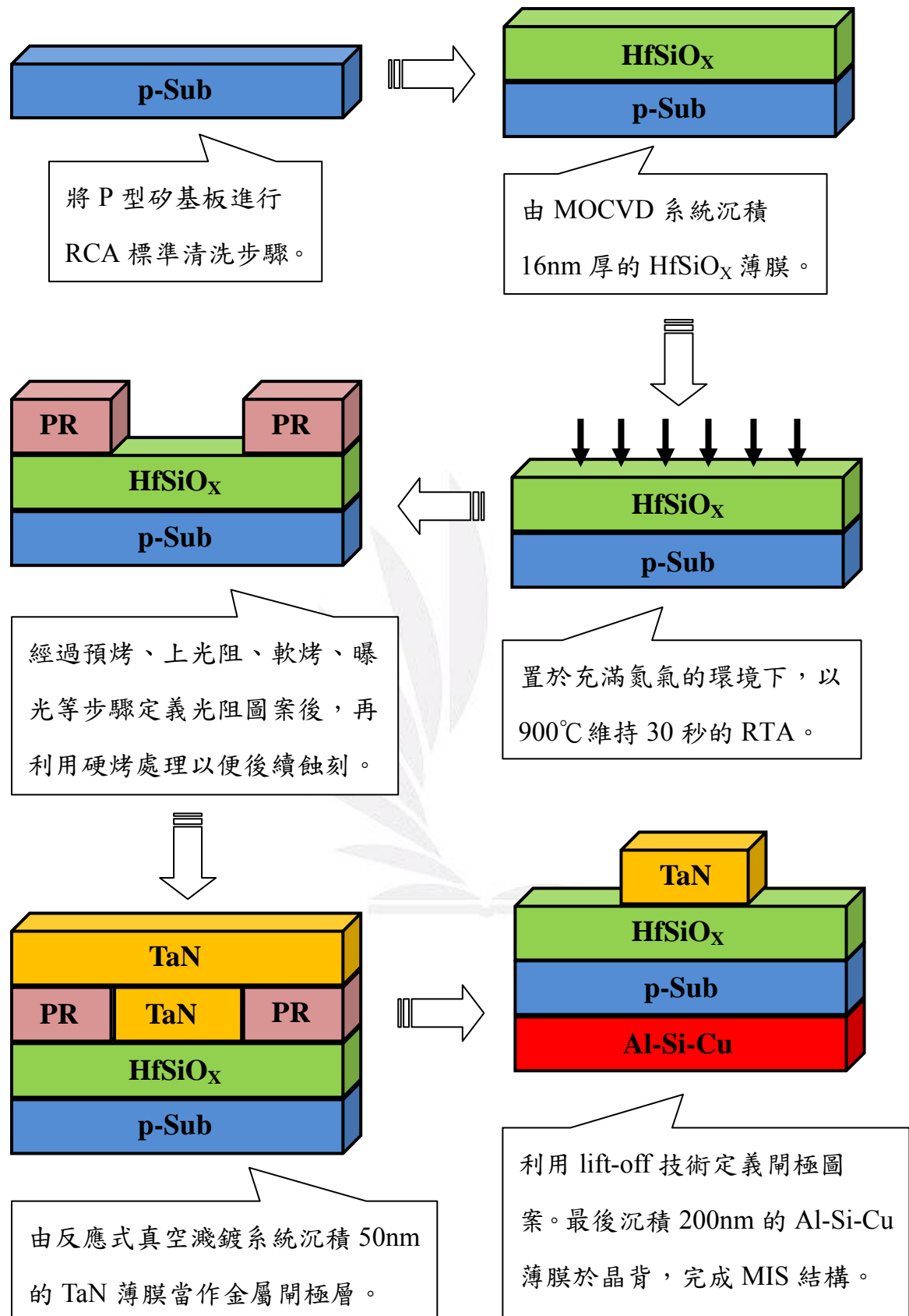
圖 3-1.2 HfSiO x MIS 結構製作流程
