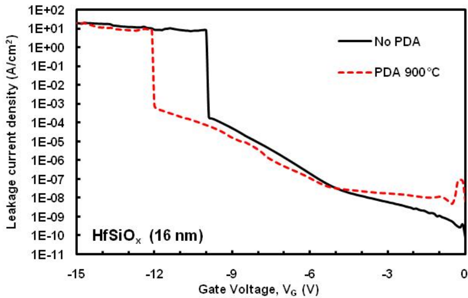
圖 3-2.1 閘極介電層 \text{HfSiO}_x (16nm)，在累積模式(accumulation mode)
