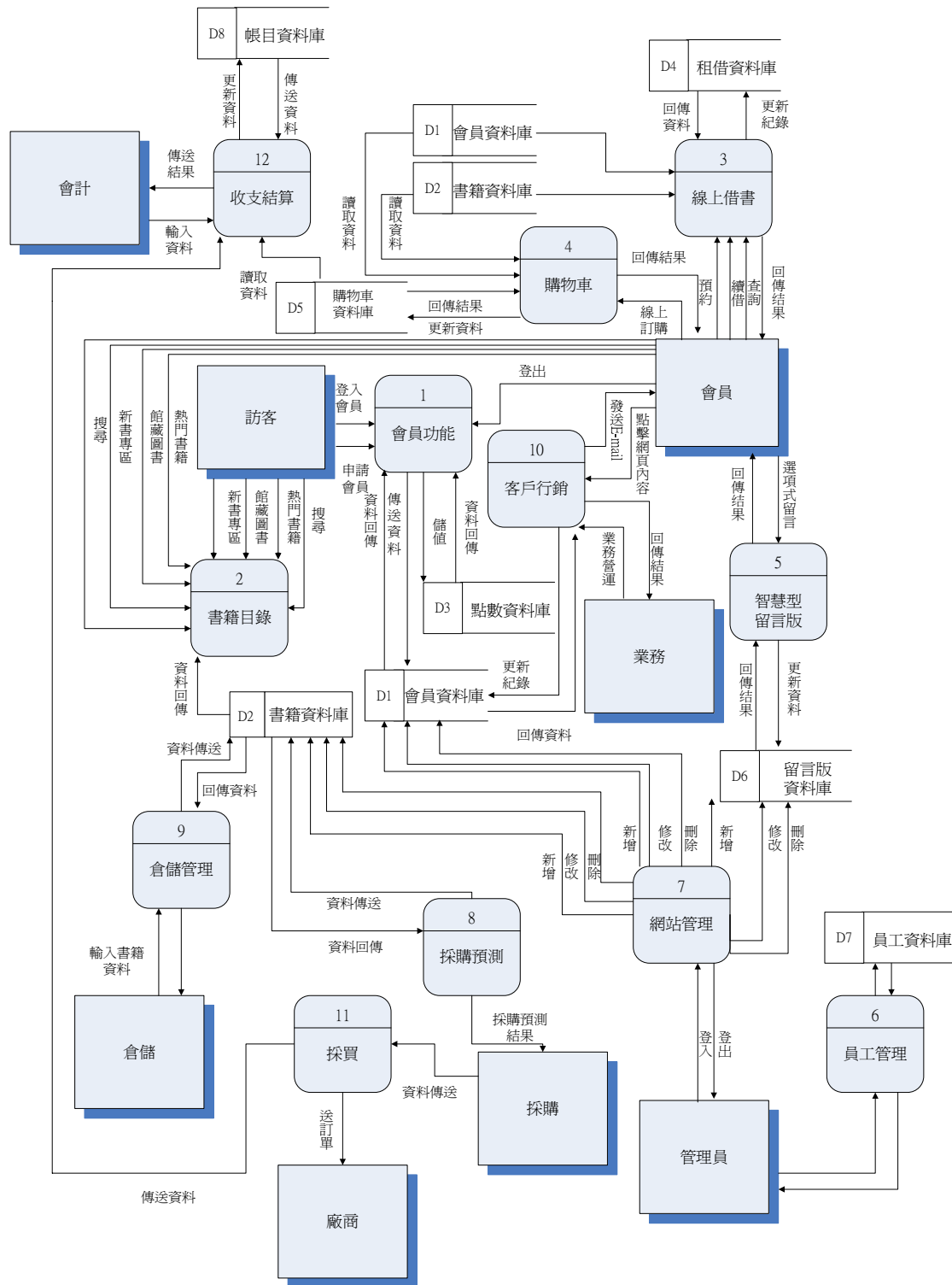
圖 3.5 圖 0
