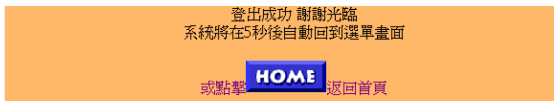
圖 4.1.2f 登出畫面
