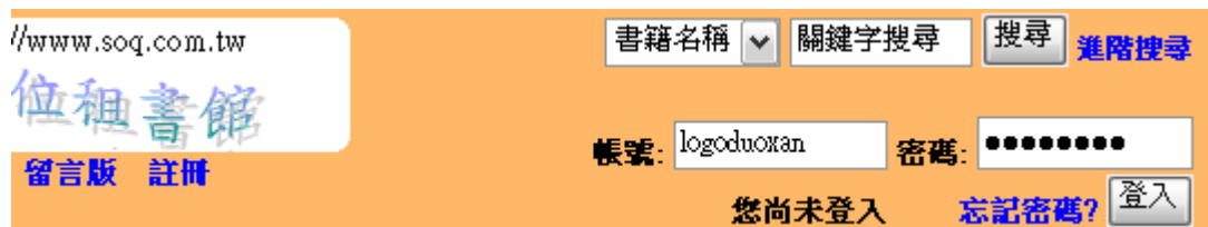
圖 4.1.2a 登入介面
