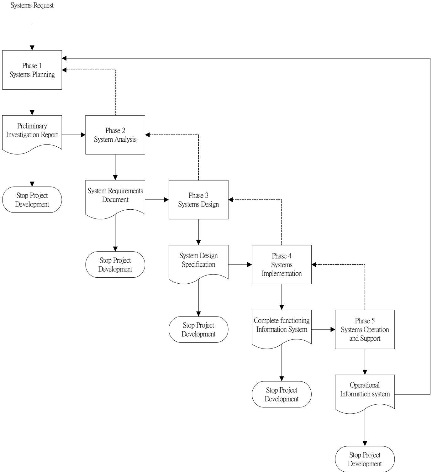
圖 3.1 SDLC 瀑布圖
